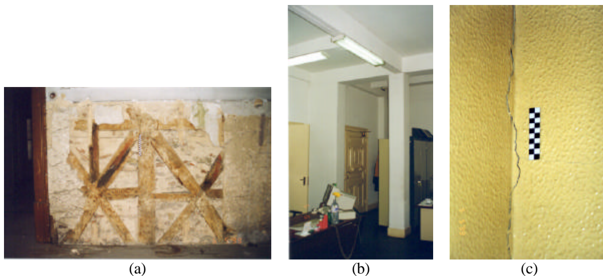
Figura 5 – Levantamento do quartirão: (a) pormenor das paredes em frontal do edifício C; (b) pormenor da estrutura do edifício G; e (c) incompatibilidade de materiais
